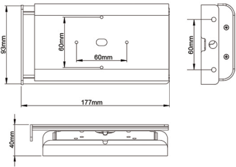
玻璃+龙骨侧装底座
