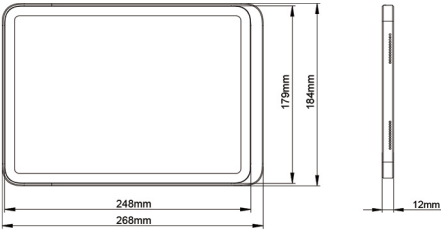
多功能平板电脑支架
