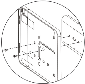
安装背板
