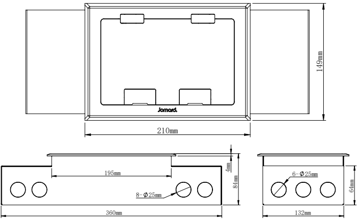
产品三视图
